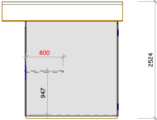
linke Seitenwand
