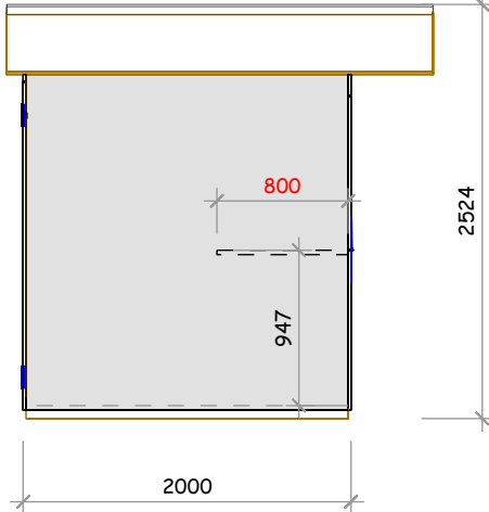
rechte Seitenwand
