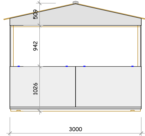
Ansicht Front
